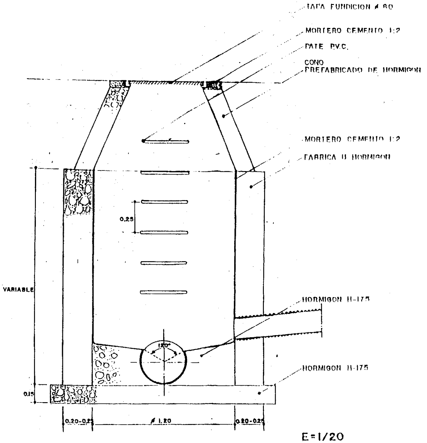
DETALLE DE POZO REGISTRABLE
