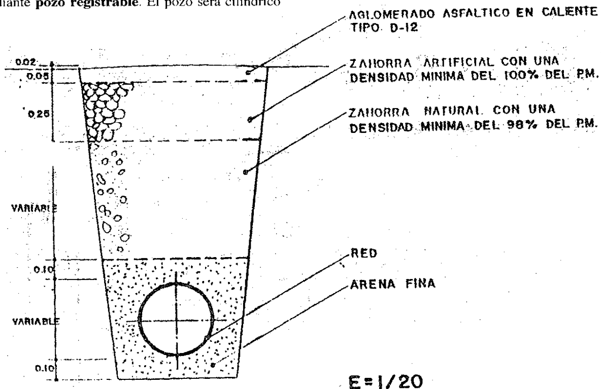
DETALLE SECCION DE ZANJA
